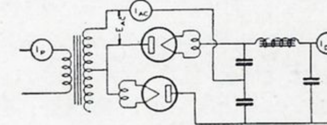
G - VOLTAGE DOUBLER RECTIFIER
